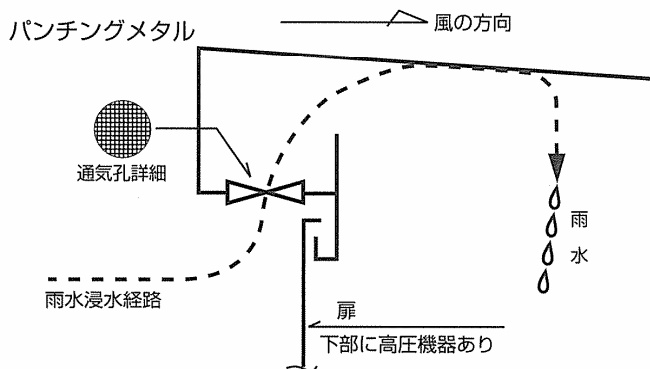
[雨水侵入図]
