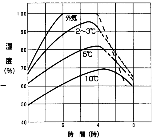
外気湿度100%持続時間に対する箱内湿度の変化
